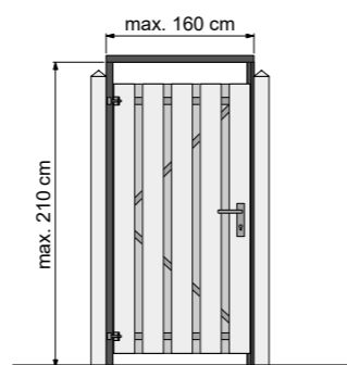
Universeel tuindeurkozijn
