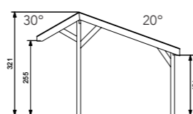
zij aanzicht
