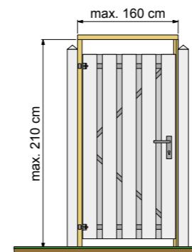
Universeel tuindeurkozijn
