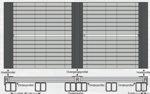
Detailtekening:
